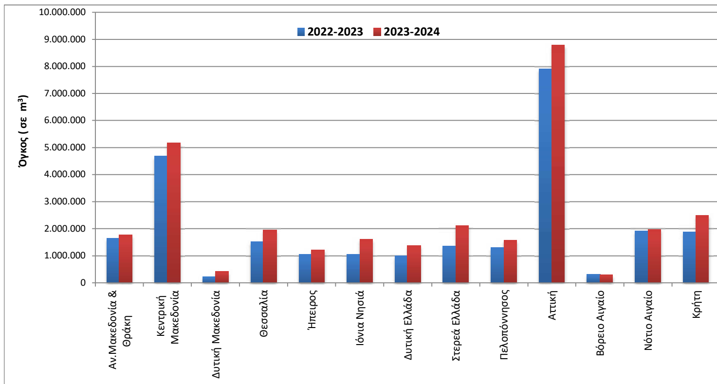
Γράφημα 2. Ιδιωτική Οικοδομική Δραστηριότητα (όγκος), κατά Περιφέρεια, για την περίοδο Ιουνίου 2022 - Μαΐου 2023 και Ιουνίου 2023 - Μαΐου 2024
